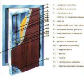
Конструкция двери
